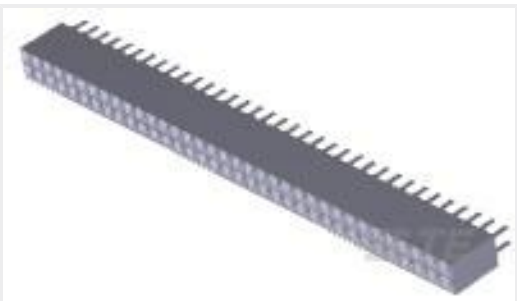
TE 产品编号3-535542-5 70 MODIV VRT DR CE 100/130
