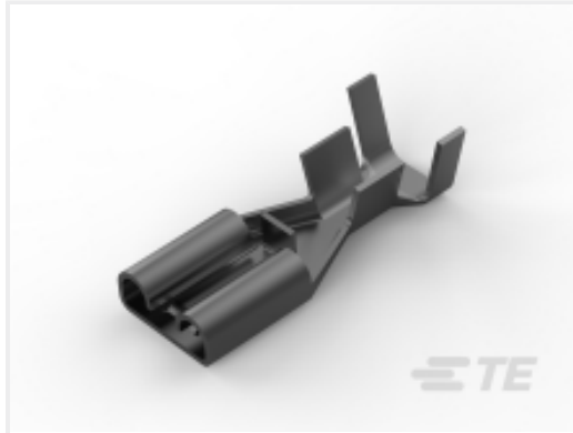
TE 产品编号 1217092-2 PL 250 TERMINAL REC 16-12 AWG TPBR
