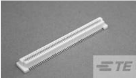
TE 产品编号 5179160-5 0.8FH,R05H.7,120,08/Sn,TR,SC,PS
