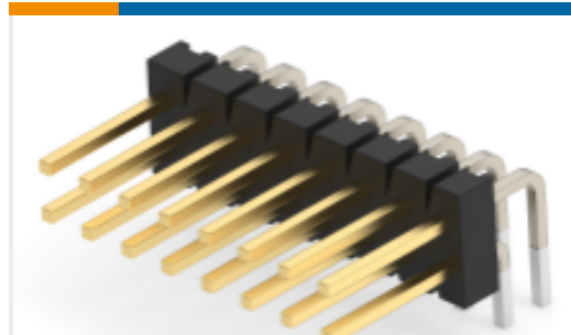
TE 产品编号 5-146309-8 16 MODII HDR DRRA B/A .100CL
