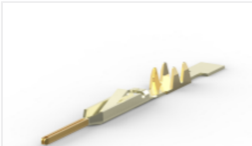
TE 产品编号 88117-9 FFC PIN CONT 15AU RL
