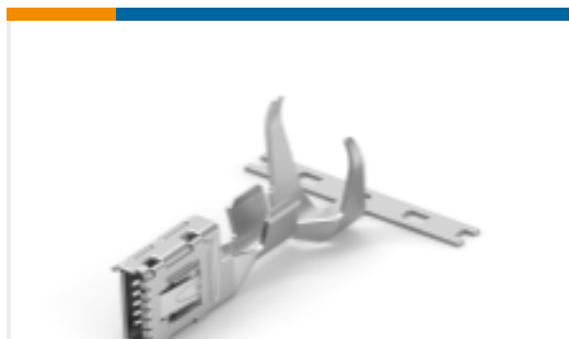
TE 产品编号1-1563844-1 MCON 9.5,CONTACT
