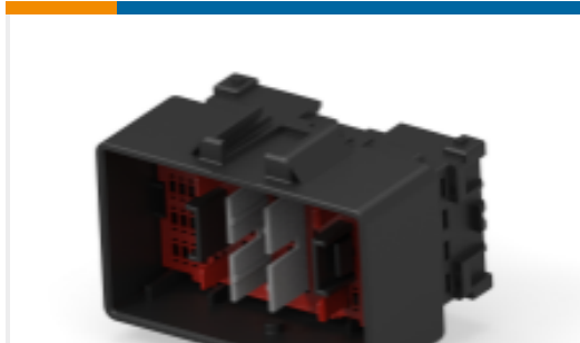
TE 产品编号2317734-1 92POS,SOC HSG,CCS,UNSLD,COD 1
