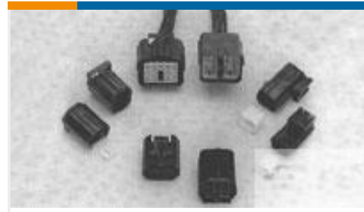
TE 产品编号 344272-1 3 WAY REC. HSG. ECONO
