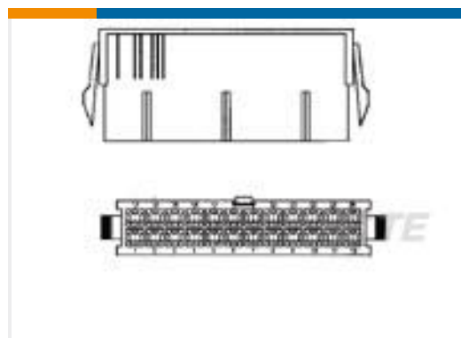
TE 产品编号1-1586018-2 12P PM PLUG VAL-U-LOK V0
