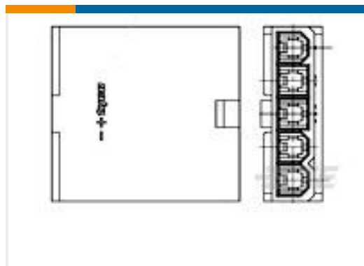
TE 产品编号1586024-5 5P S/R FH PLUG VAL-U-LOK V2
