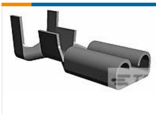
TE 产品编号60487-1 187 FASTON REC 18-16 AWG BR
