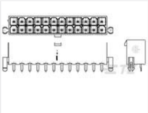
TE 产品编号1586039-2 2P VAL-U-LOK VRT HDR W/P V2
