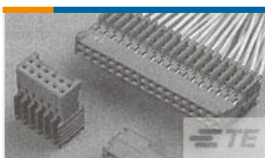
TE 产品编号 1-281792-5 PLUG HE14 IDC 180 2X15 P AWG 28-26
