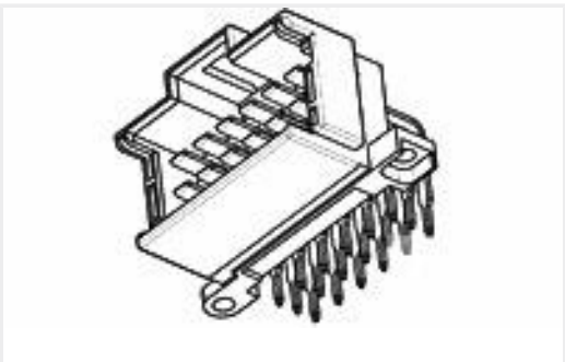
TE 产品编号966140-2 MESSERLEISTE 15P
