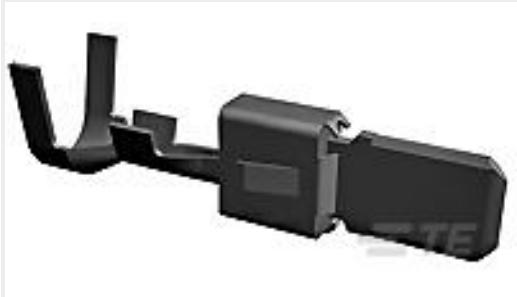
TE 产品编号1-962919-2 TAB 5.8x0.8 CONTACT CS SWS Ag
