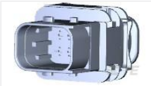
TE 产品编号1-1564512-1 8POS,TAB 1.6X0.6,TAB HSG,ASSY
