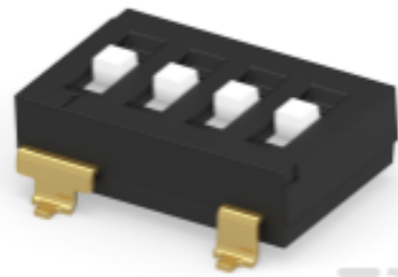
TE 产品编号 1-2319747-6 TRI-STATE DIP 4P G RAISED T&R
