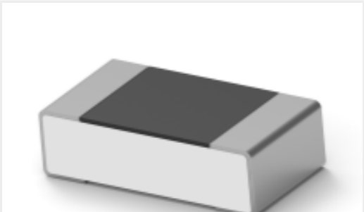
TE 产品编号4-2176371-8 RQ 0603 14K3 0.1% 10PPM 5K RL
