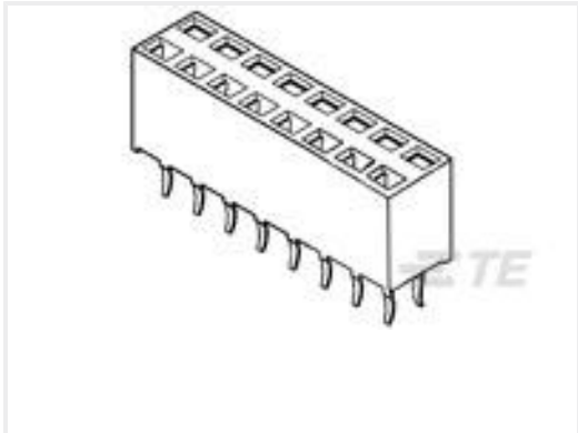
TE 产品编号4-1241852-5 HV100 CONN2X5P VERT
