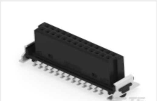
TE 产品编号154806-E SMCB 26 F AB VV 7-13 CL * H007 137 E002
