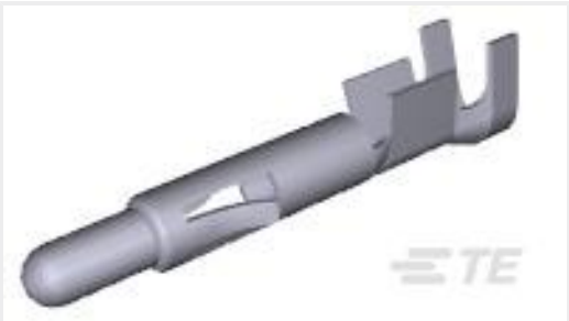
TE 产品编号350547-6 UMNL PIN 20-14 AU/PHBZ L/P
