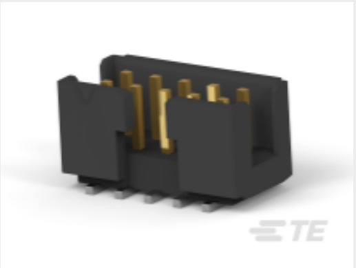
TE 产品编号 1-2842279-4 14P,2MM,SHRD HDR,DRVVT,SMD,0.38 AU,TR W/CP
