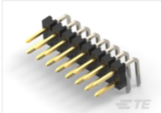
TE 产品编号 1-2823136-4 14P,2MM,BRK HDR,DRRT,2.8,0.38AU, TB
