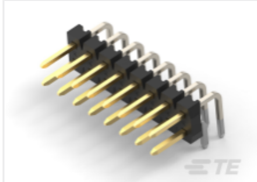
TE 产品编号 1-2823134-4 14P,2MM,BRK HDR,DRRT,2.2,0.38AU, TB
