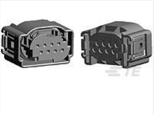
TE 产品编号2-1534229-1 8POS MQS REC COD B
