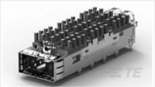
TE 产品编号1888971-1 Cage Assy Thru Bezelw/LP San, QSFP
