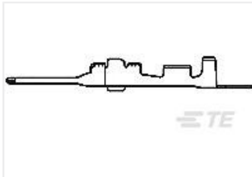
TE 产品编号917067-6 040-2 TAB CONT S GOLD 22-18
