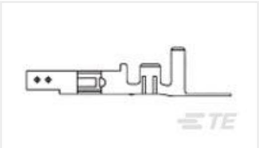
TE 产品编号794956-1 VAL-U-LOK SKT BR SN 22-18AWG
