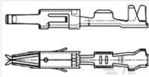
TE 产品编号965914-2 MT3 REC 1.6 Contact SRC Sn
