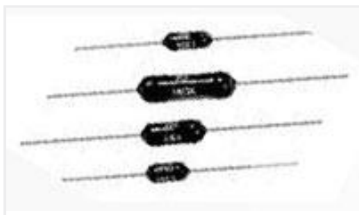
TE 产品编号9-1879685-0 H8 105K 0.1% 50PPM
