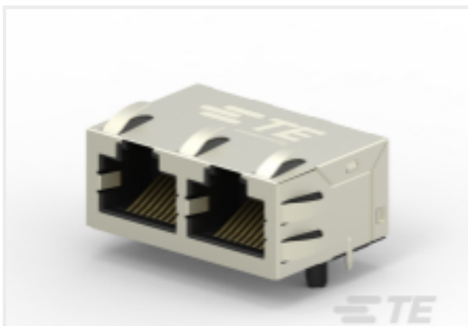
TE 产品编号5-2301996-1 RJ45 JACK INT.MAG. 10/100 1X2 INV.
