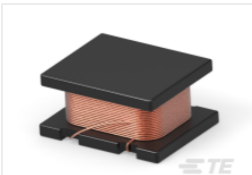
TE 产品编号1-2176638-4 3627C 322515 100UH 20%
