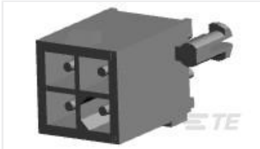
TE 产品编号1-770174-0 04P MINI-UMNL ASSY VO SNNI*
