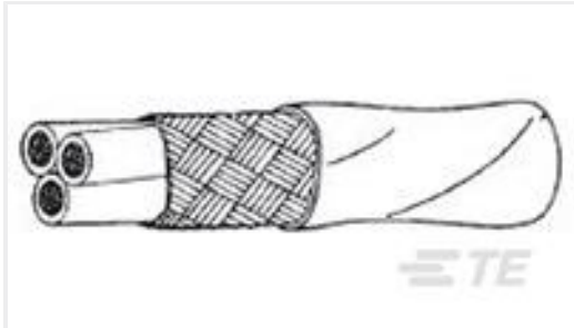
TE 产品编号316062-005 55A1131-22-2/4/6-9
