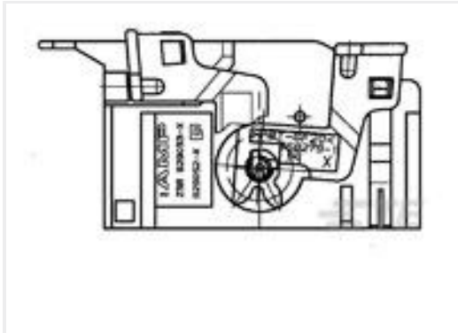
TE 产品编号929053-1 MQS ABDEKA M.HEB32P
