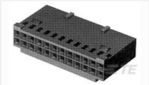
TE 产品编号87631-5 10 MODIV HSG COMP DR .100 POL
