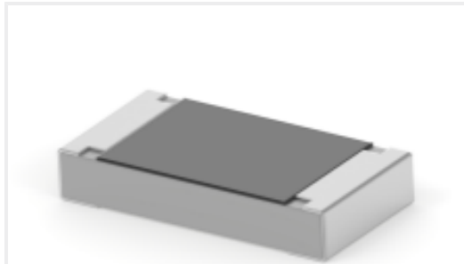
TE 产品编号1-2176344-7 CRGCQ 1206 470R 5%
