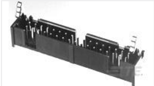
TE 产品编号1761608-7 IDC LOW PRO HDR 20P VERT SHT L
