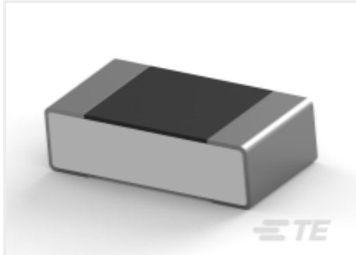
TE 产品编号9-2176370-2 RQ 0603 3K83 0.1% 10PPM 5K RL
