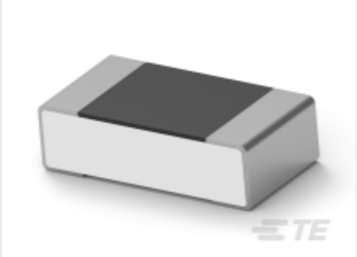
TE 产品编号3-2176371-1 RQ 0603 9K53 0.1% 10PPM 5K RL
