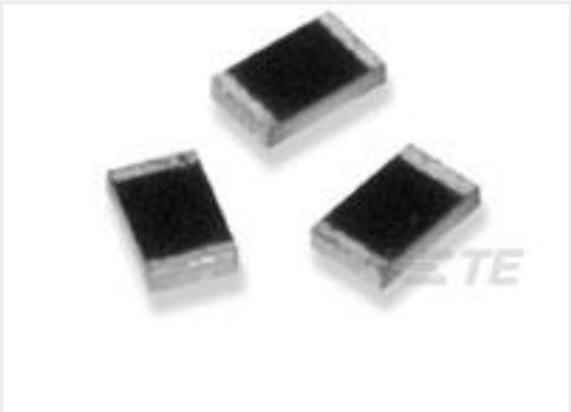
TE 产品编号1625868-1 RP 2A 0.25W 11K 0.1% 25PPM 1K RL
