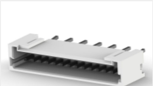
TE 产品编号3-292207-4 MINI CT SGL DIP V 14P BLACK
