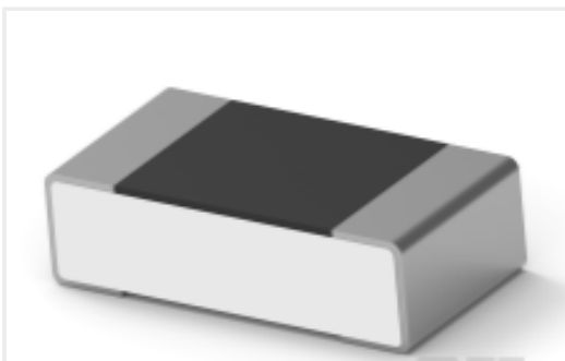
TE 产品编号8-2176366-9 RQ 0603 3K57 0.1% 10PPM 1K RL
