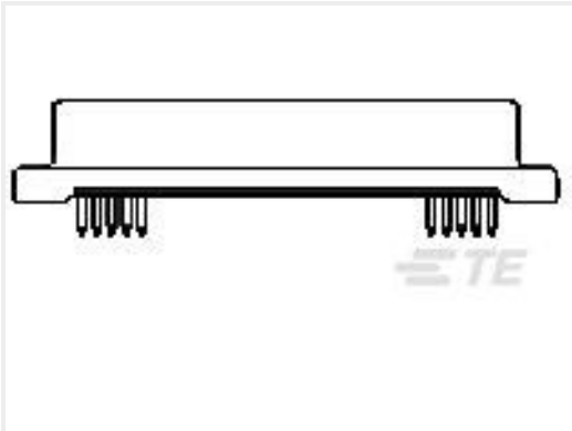
TE 产品编号5173279-3 MINI MITE PLUG ASSY 50P (V)
