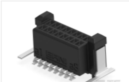
TE 产品编号294001-E DRCB 0,80 16 F SMD F4 137 E009 094 GU-H
