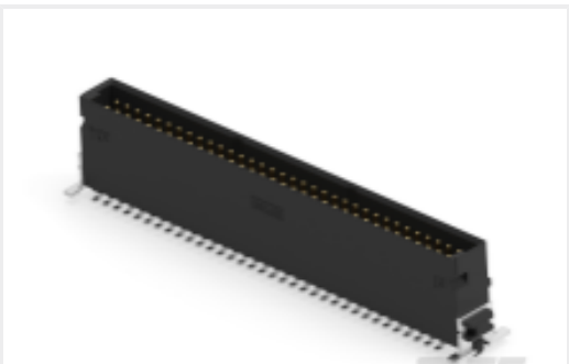
TE 产品编号234209-E SMCQ 68 M AB VV 8-23 CL * H007 137 E005
