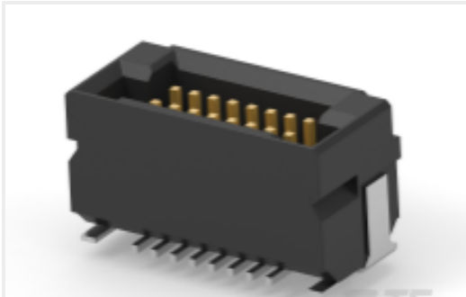
TE 产品编号454928-E DRCQ 0,80 16 M 2 SMD M2 137 E009 176 GU-
