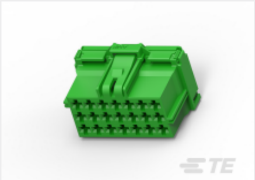
TE 产品编号CAT-AM705-CH8173 AMP 非密封连接器外壳
