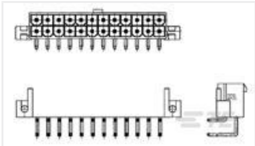
TE 产品编号1-1586044-8 18P VAL-U-LOK R/A HDR SCRMT V0
