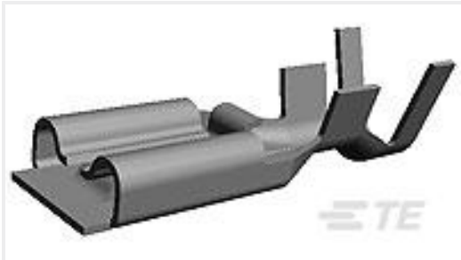
TE 产品编号173724-5 PL EX 187 REC 20-14AWG PTPB
