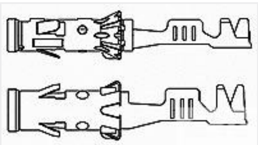
TE 产品编号1-929974-4 2,5MM SWS REC.CONT.
