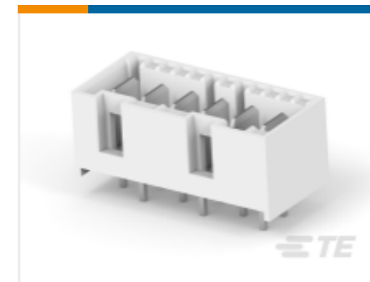
TE 产品编号 6-1971845-6 6P, RAST 5 Tab Header, THV
