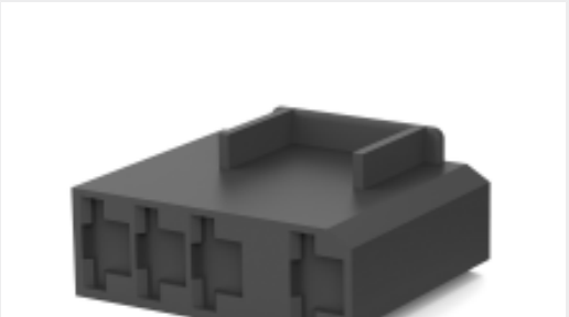
TE 产品编号1-520987-4 250 FASTON HSG.,REC.,4 POS,BLACK
