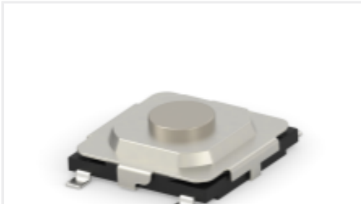
TE 产品编号 2337237-3 TACT MINI GW 5.2X5.2X1.5 160GF
