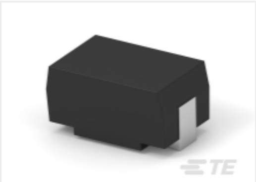
TE 产品编号CAT-C339-SM1A SMD 功率电阻器：7 瓦特，.10-500 欧姆
