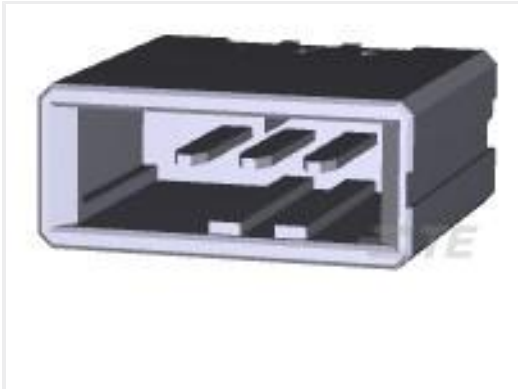
TE 产品编号1-178313-2 DYNAMIC D3100 HDR V 3P ASSY PdNi & Au PL
