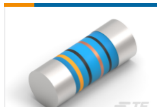
TE 产品编号3-2176316-6 MELF SMA_A 82K 0.1% 15PPM 0207 1W
