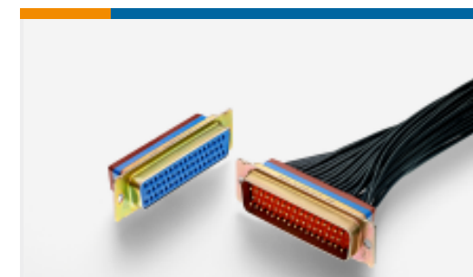
TE 产品编号1-2157481-3 AMPLIMITE IP67, SZ3, 109, 25 POS, RCPT
