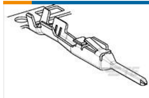
TE 产品编号1674742-1 025 TH TAB CONTACT
