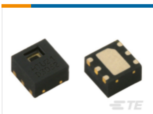
TE 产品编号HPP845E031R1 I.C 21D RH/T B1500
